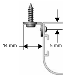
ODD geschroefd
