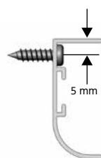
IDD geschroefd
