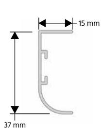
Profiel geleiding
